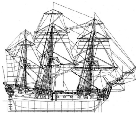
66-пушечный линейный корабль «Св. Евстафий Плакида»
