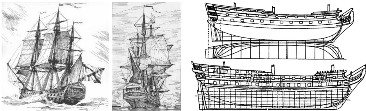
66-пушечные линейные корабли «Ростислав» (слева) и «Не тронь меня» (в центре). С гравюр XVIII в. Справа – чертежи корпусов 66-пушечных линейных кораблей «Трех Святителей» (наверху) и «Иануарий» (внизу)
