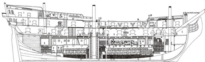
66-пушечный линейный корабль «Трех Иерархов»: общий вид (наверху) и разрез корпуса (внизу)
