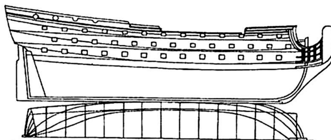
Чертеж 80-пушечного линейного корабля «Кир Иоанн»
