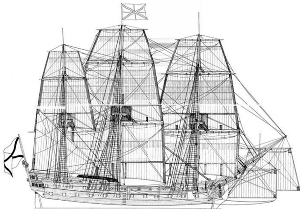
66-пушечный линейный корабль «Св. Евстафий Плакида»
